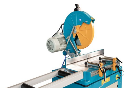
La tête de scie peut s'incliner des deux côtés jusqu'à 45°
